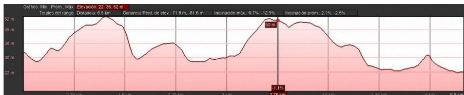
Fig 7. Corte Transversal (calles 18 de julio y Joaquín Suárez). Fuente: Google Earth, 2020
