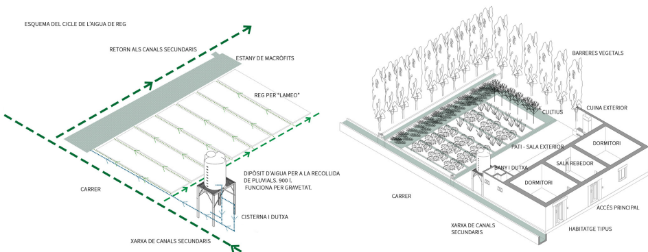
Fig. 16. Esquema del cicle de l'aigua de reg. Font: Elaboració pròpia
